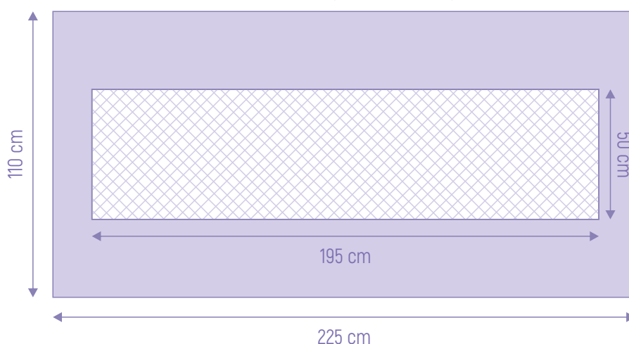
Základní rozměry komplexního krytí
